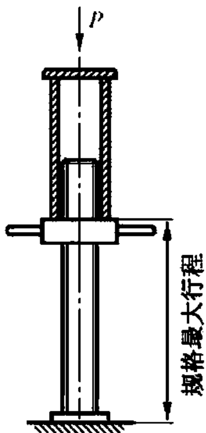
图 6 可调支座抗压强度试验示意图
